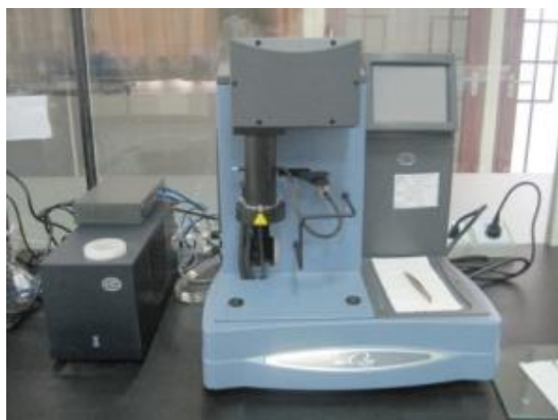
TGA热重分析仪 Thermal Gravity Analyzer
