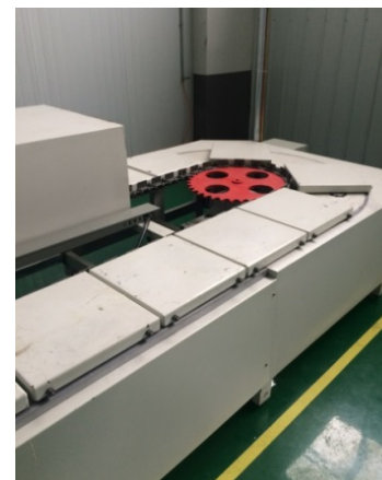
加热烘道 Heating oven
